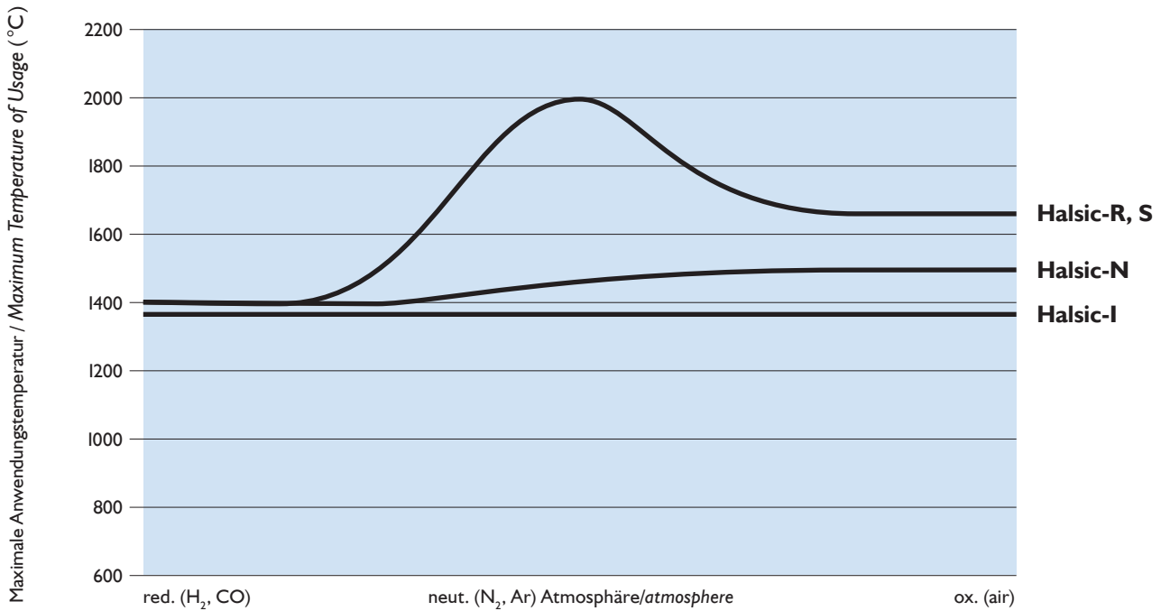
Maximale Beständigkeitstemperaturen unter den angegebenen Atmosphärenbedingungen für Siliziumkarbid-Werkstoffe (Halsic) Maximum operating temperatures for the different atmospheres given for silicon carbide materials (Halsic)
